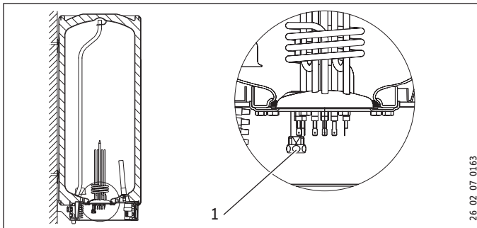
1 Kappe Entleerung G 1/2
