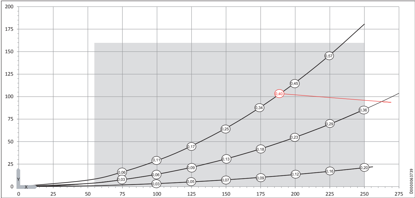
LWZ 180 / LWZ 180 Enthalpie
