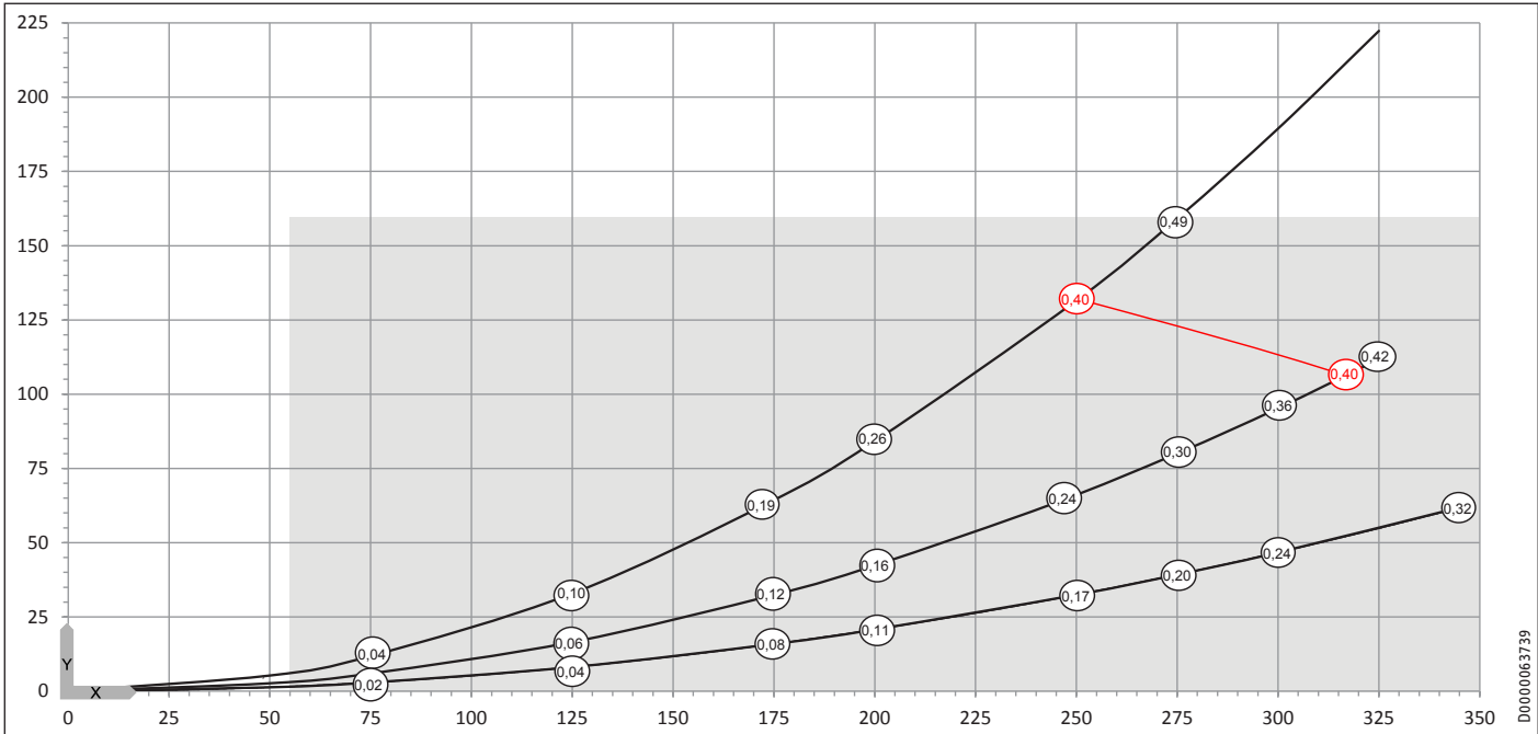
LWZ 280 / LWZ 280 Enthalpie
