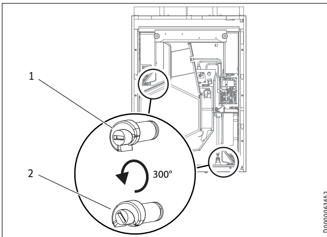
1 Upnutý excentrický čep (drážka vodorovně).
