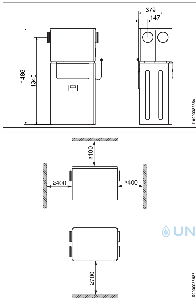
Rysunek ustawienia z nasadką dźwiękochłonną
