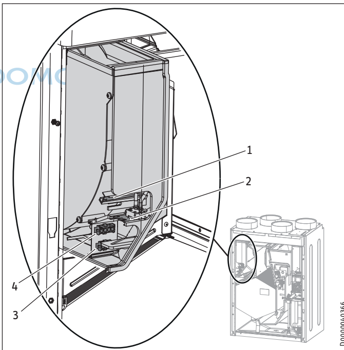
1 Připojení snímače teploty
