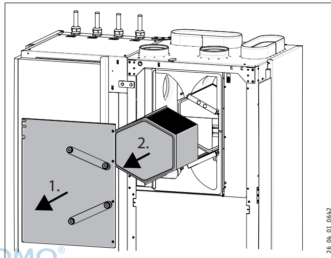
1 Horní čelní kryt
