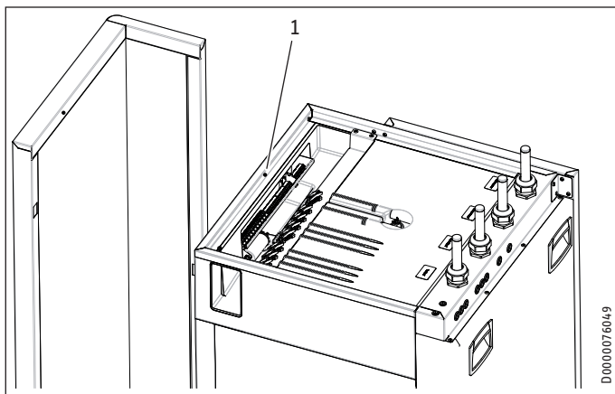
1 Šroub pro upevnění přední stěny
