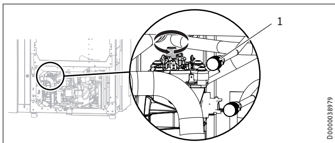
1 Odvzdušňovač deskového tepelného výměníku
