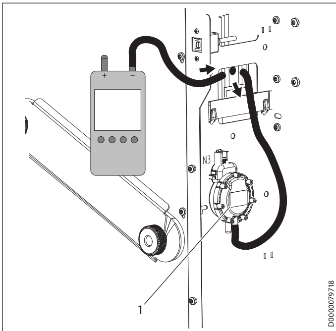
1 Differenzdrucksensor
