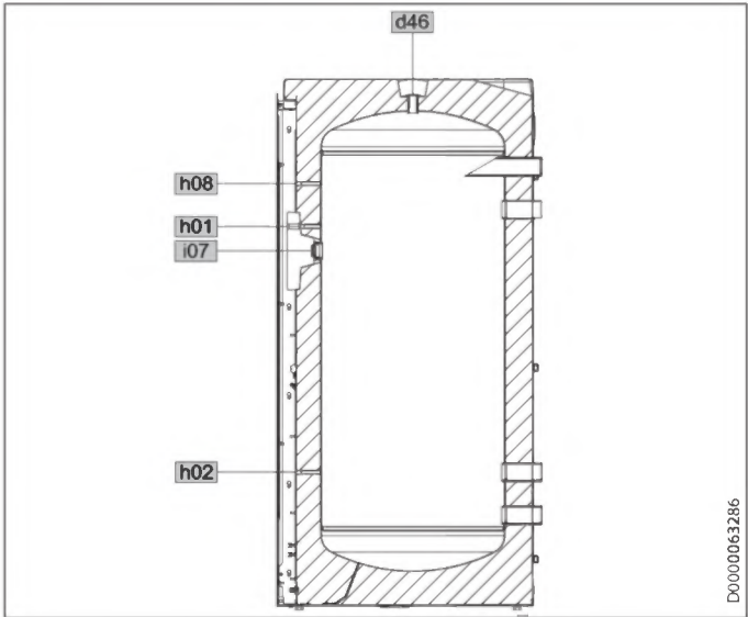
Другие размеры и подключения
