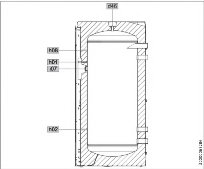
Autres cotes et raccordements
