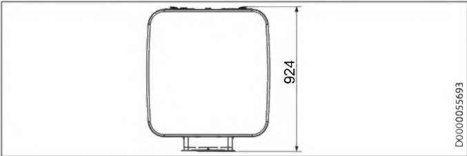
Вид спереди (со съемной рамой)
