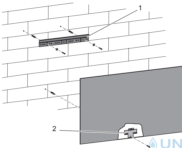
1 Wandkonsole 2 Haltewinkel
