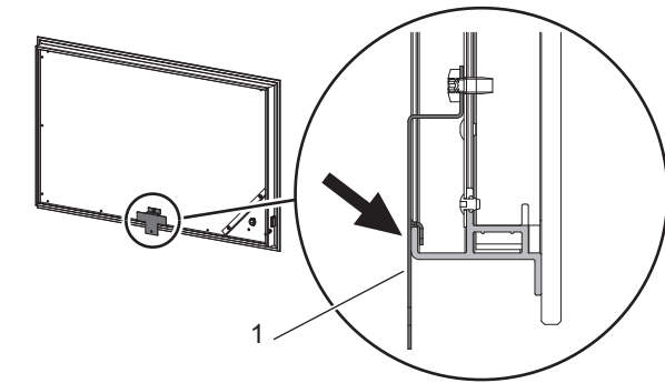
1 Haltewinkel
