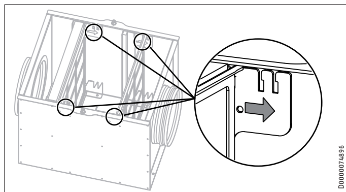
2 Filtrerrahmen
