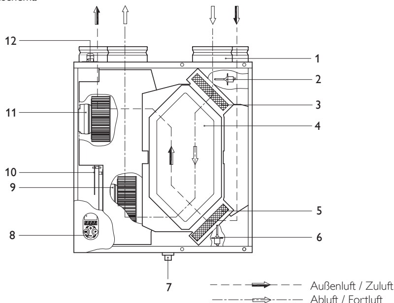
Funktionsschema
