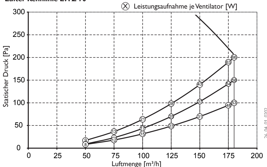
Lüfter-Kennlinie LWZ 70
