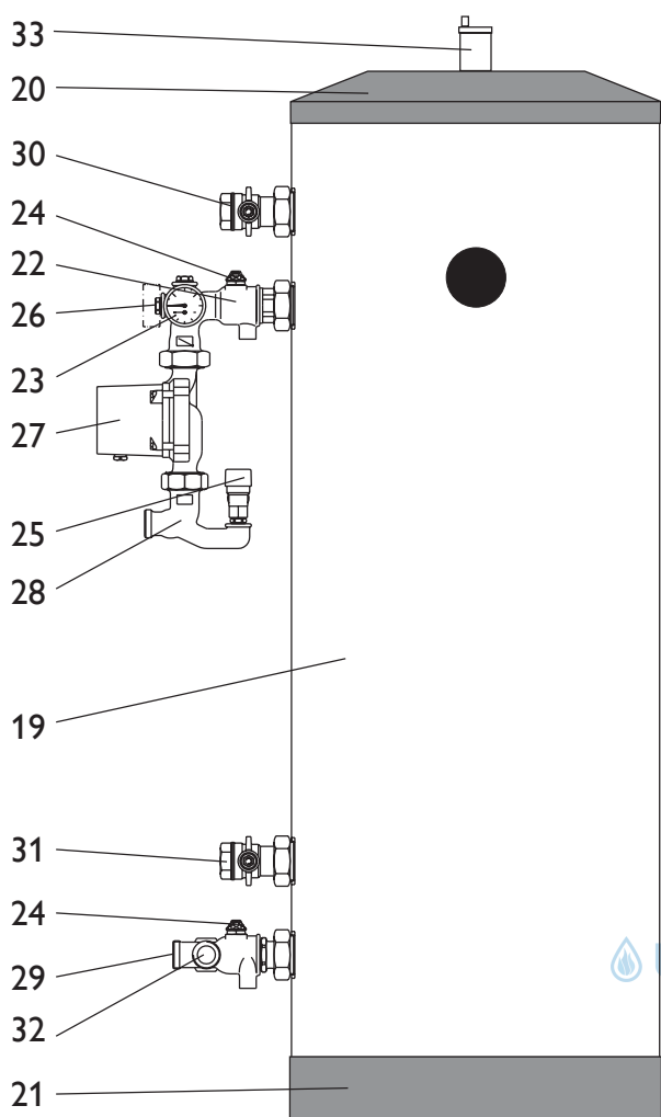
SBP 200 E mit WPKI 3
