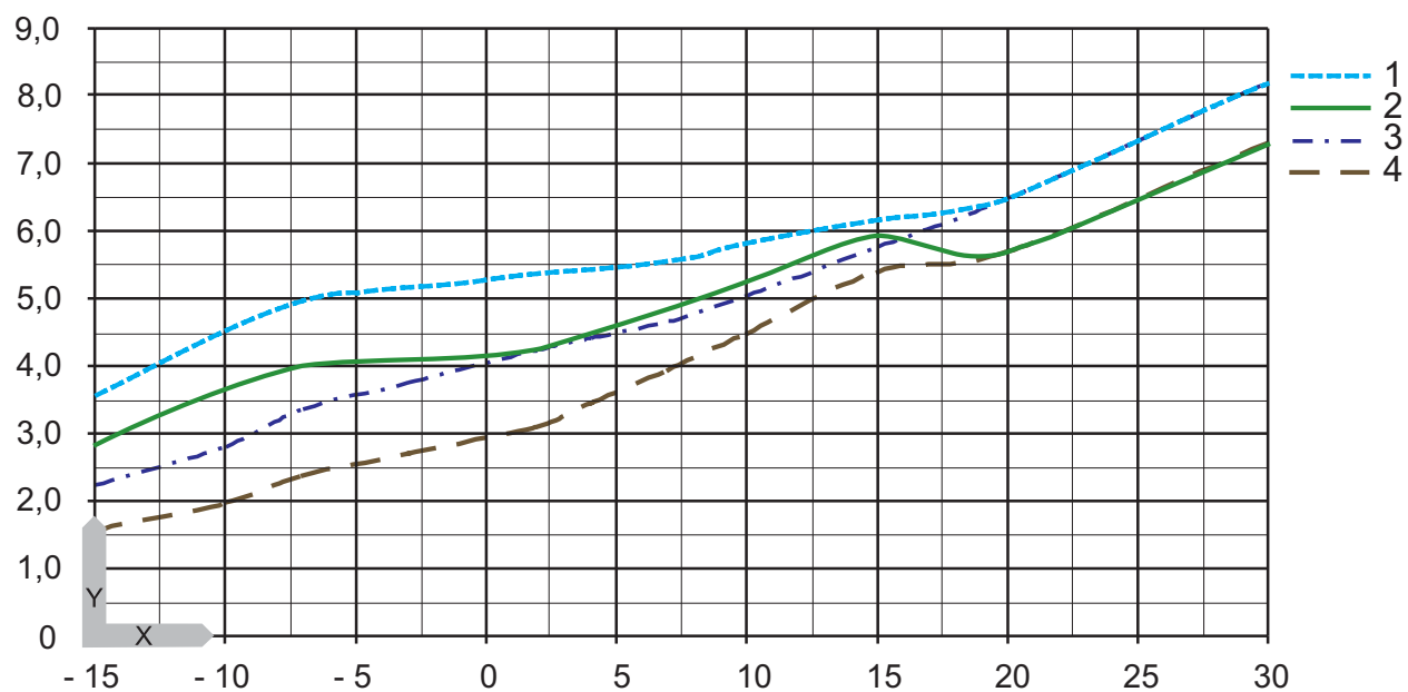
LWZ 303 SOL teljesítménydiagram
