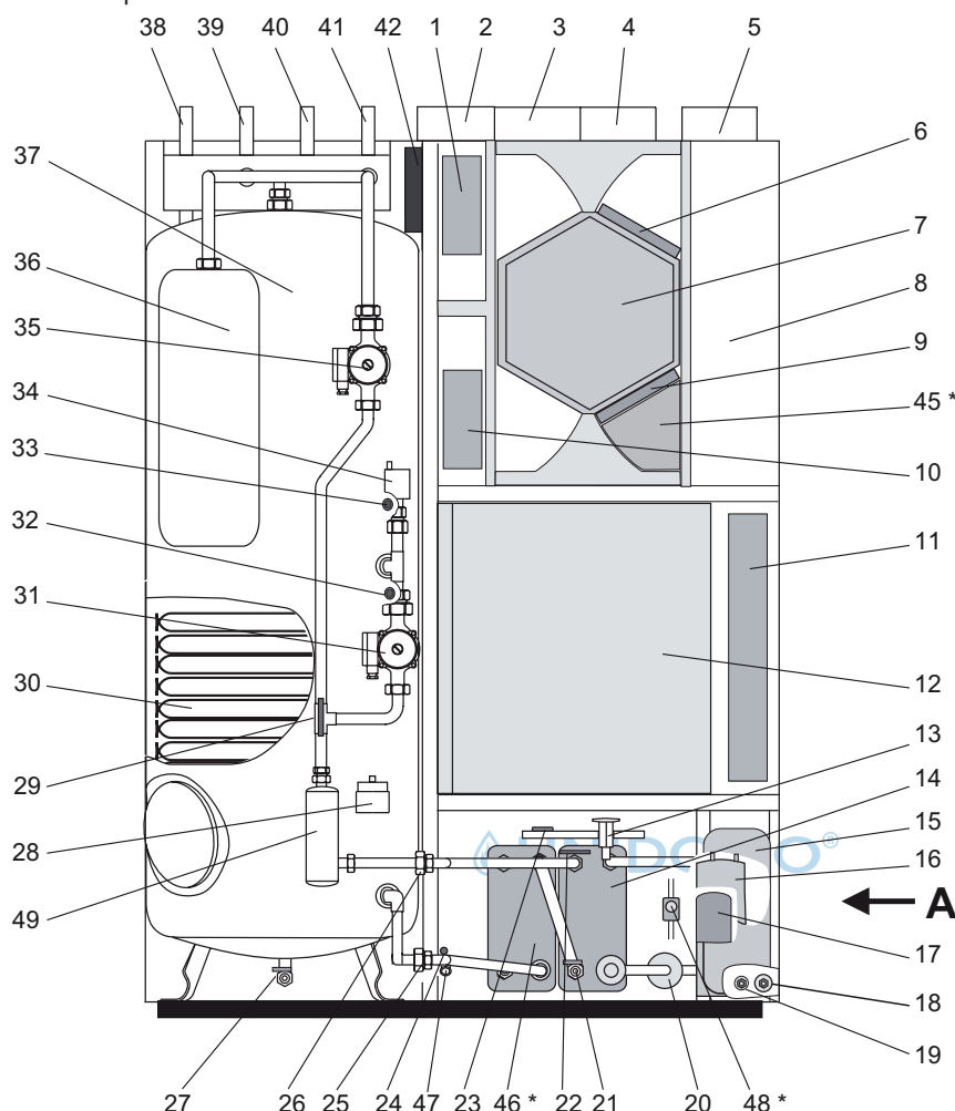
A berendezés felépítése
