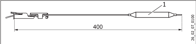
1 Thermostaat-sensor dompeldiepte
