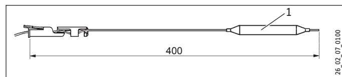
1 Temperaturregler-Fühler
