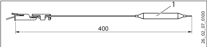
1 Датчик регулятора температуры
