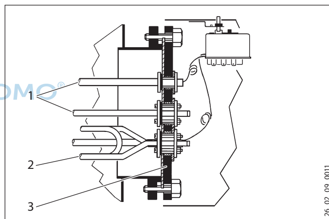
1 Защитная трубка 2 Нагревательный элемент 3 Фланцевая пластина
