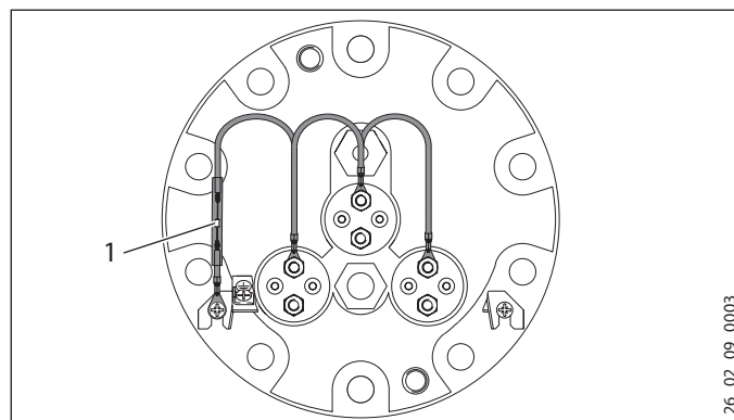
1 Антикоррозионный резистор 390 Ом
