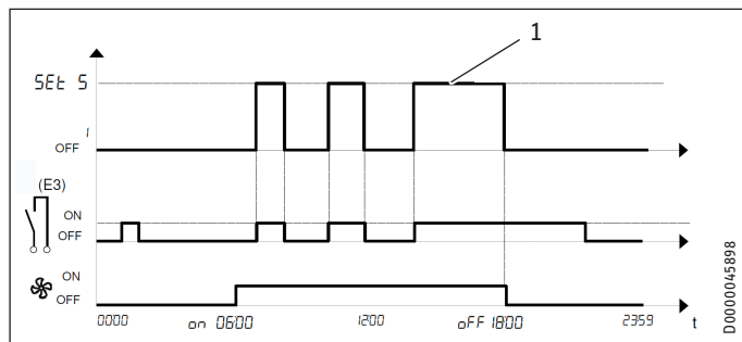
1 Kennlinie Lüfterdrehzahl
