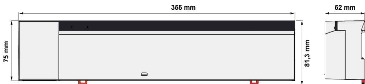
Rollenabmessungen 12-Zonen Basisstation:
