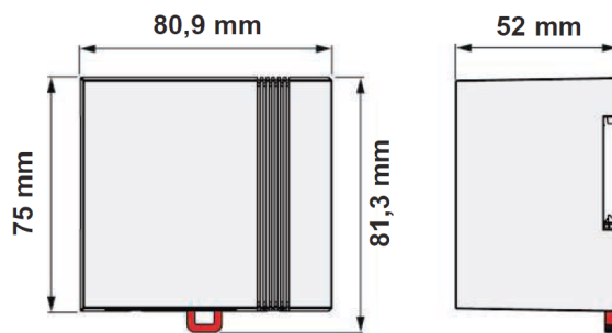
Abmessungen Trafo:
