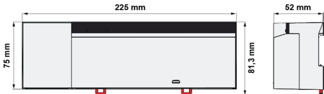
Abmessungen 4-Zonen Basisstation:
