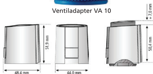
Abmessungen
