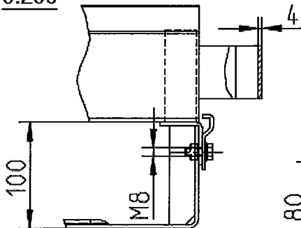
Detail B 0.200
