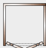
Flügeltür, 2-teilig Einstiegsbreite ca. 650 mm
