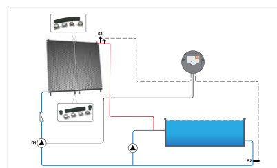
Betrieb mit eigener Pumpe, Schwimmbadpumpe und Roth Solarregelung E* SW in den Filterkreislauf integriert
