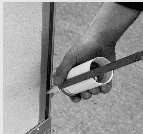
Silikon beim Aufklappen der Wandplatten in die Scharnierprofile einbringen Assurer l'étanchéité des profils charnières. Filling silicone into the hinges while opening the wall tiles
