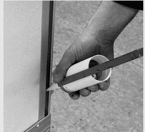
Silikon beim Aufklappen der Wandplatten in die Scharnierprofile einbringen Assurer l'étanchéité des profils charnières. Filling silicone into the hinges while opening the wall tiles
