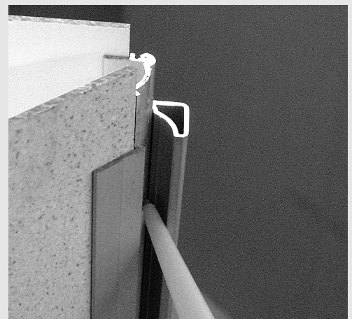
Scharnierprofile in voller Länge eindichten L'étanchéité des profils charnières est à réaliser comme sur la photo et sur toute la longueur. Sealing of hinges in full length
