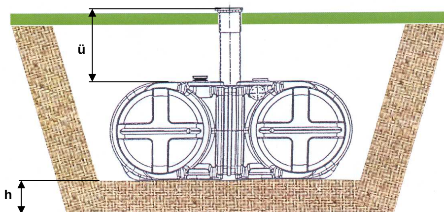
Skizze 1: Abmessungen Baugrube f. Sammelgruben Twinbloc
