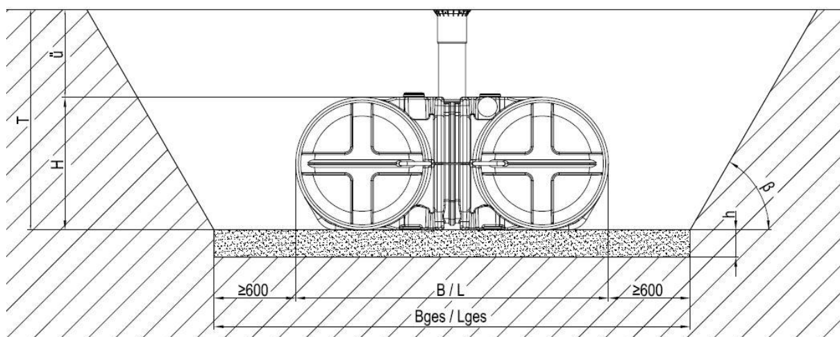
Abbildung 1: Baugrube
