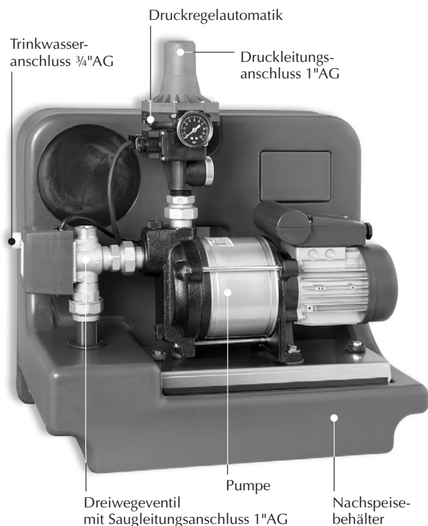
Bild 4 Aufbau
