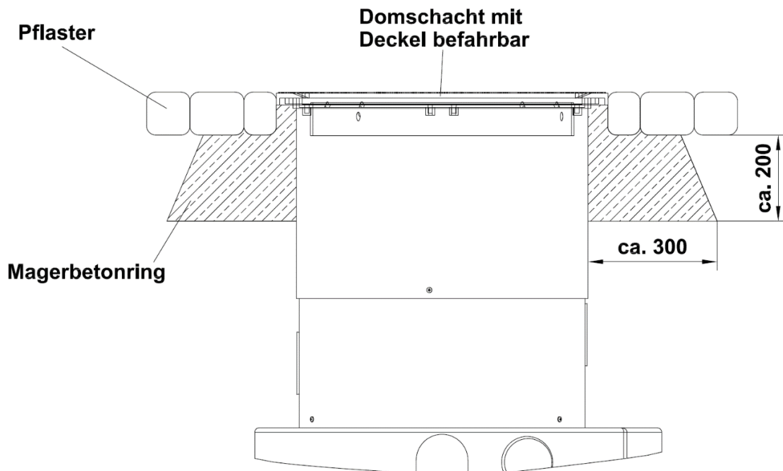
Abbildung 5: Pkw-befahrbarer Teleskop-Domschacht
