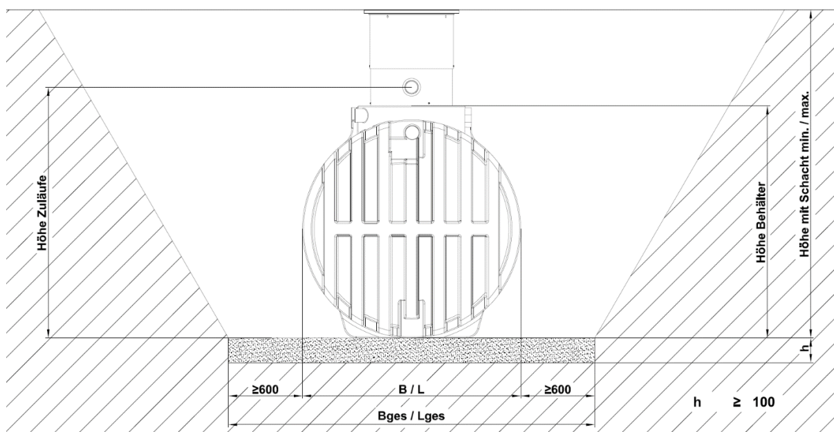
Abbildung 1: Baugrube
