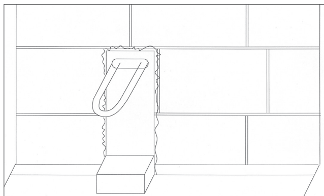
Einbau direkt auf Rohfußboden
