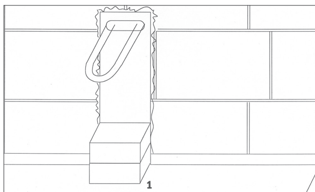
Einbau mit Unterbau auf Rohfußboden
