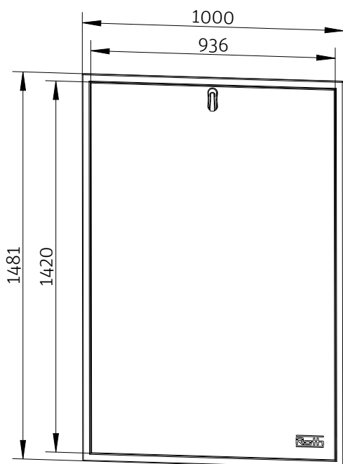
Roth FlatConnect Tür und Rahmen UP Größe 1 Mat.-Nr.: 1150011329
