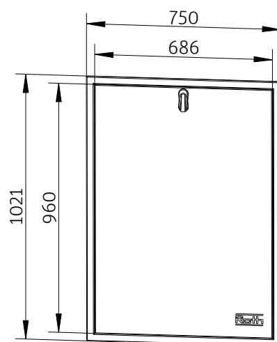
Roth FlatConnect Tür und Rahmen UP BM Mat.-Nr.: 1150011325
