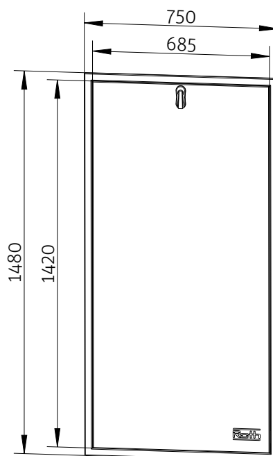
Roth FlatConnect Tür und Rahmen UP Größe 0 Mat.-Nr.: 1150011327
