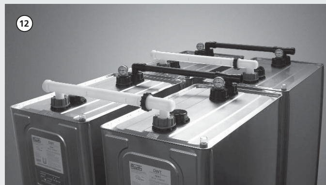
Montageschritte der Leitungen für jede Tankreihe wie auf den Bildern 2, -3, -5, -6, -7, -8 gezeigt wiederholen, außer... Repeat installation steps for the lines for each tank row as indicated in images 2, -3, -5, -6, -7, 8., except... Reprendre les étapes de montage des conduites pour chaque série de réservoirs comme le montre les dessins 2, -3, -5, -6, -7, -8, excepté... Montageschappen van de leidingen voor elke tankrij herhalen zoals afgebeeld in afb. 2, 3, 5, 6, 7, 8, behalve...
