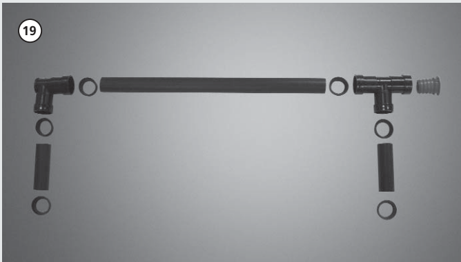
Entlüftungs-Sammelrohr vormontieren und... Pre-assemble ventilation manifold and... Prémonter le tube collecteur de purge et... Ontluchttings-verzamelbuis vormonteren en ...
