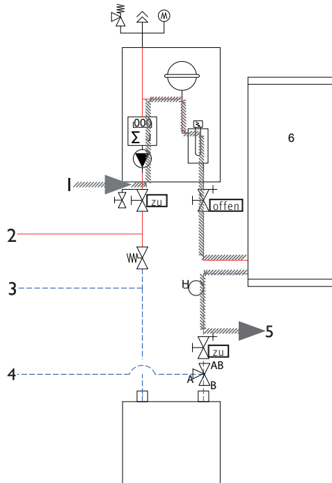
Beispiel Reihenspeicher:
