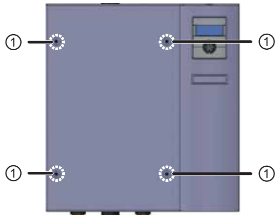
1 Schnellverschlusschrauben
