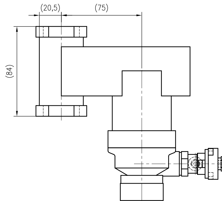
UNIDOMO® Front view
