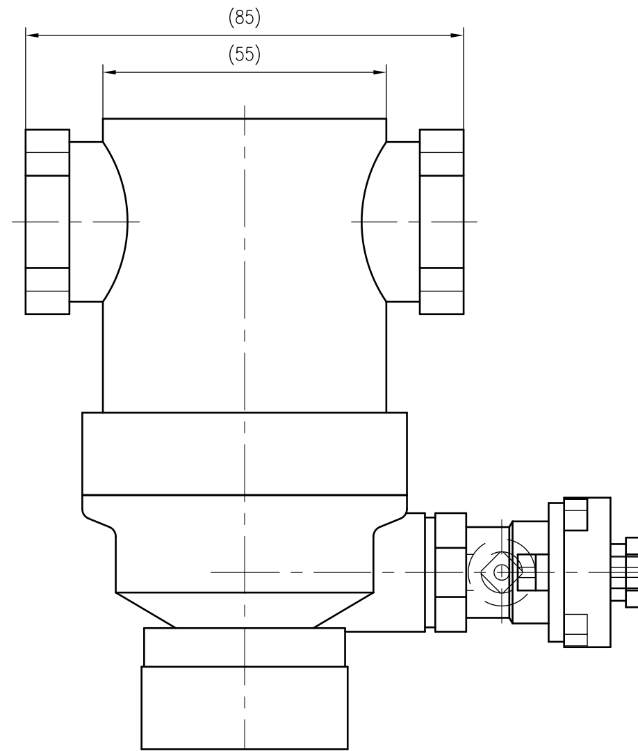
UNIDOMO® Front view
