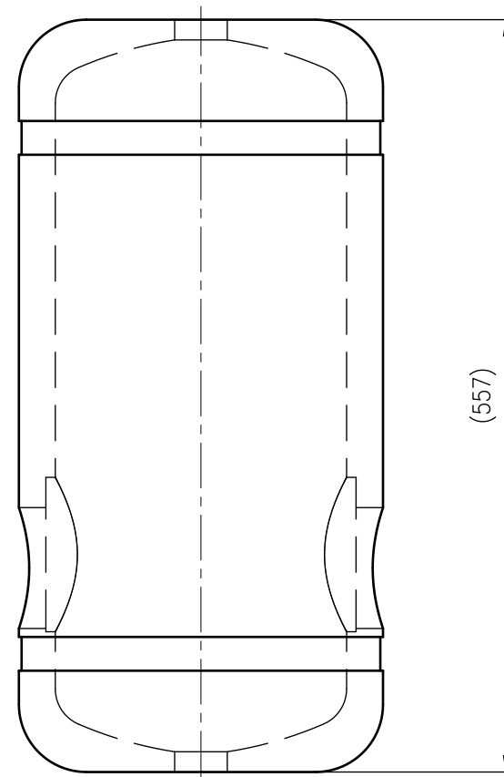
UNIDOMO® Front view
