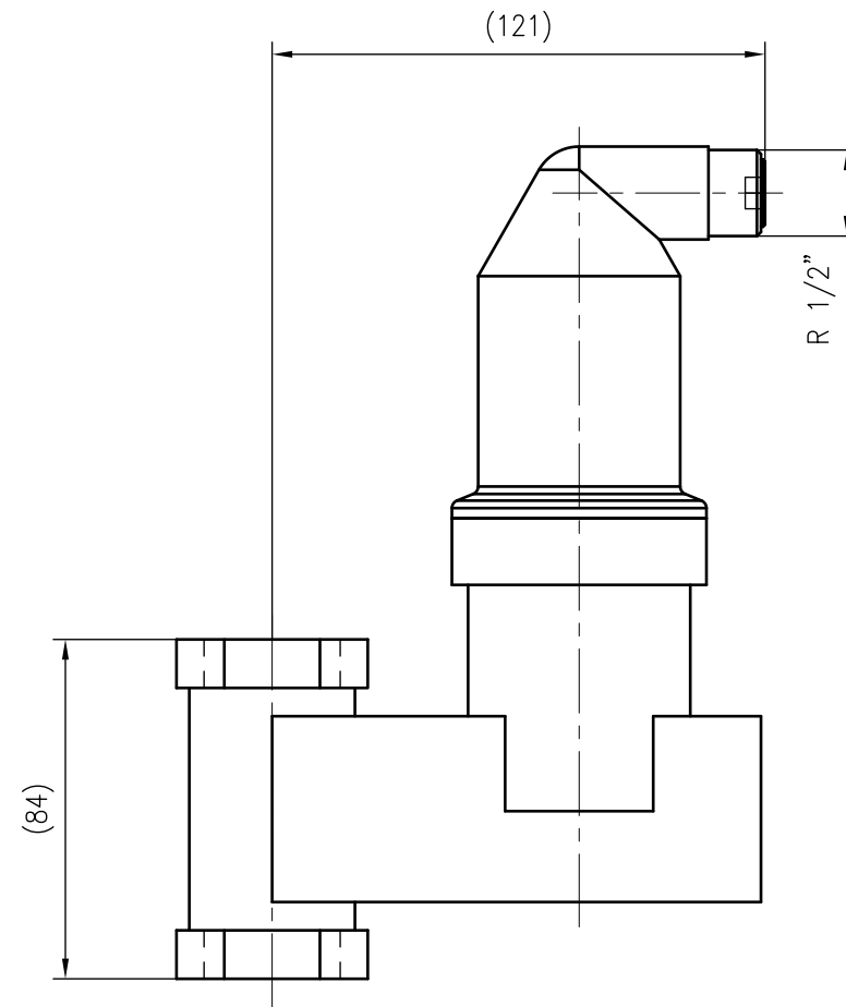
UNIDOMO® Front view
