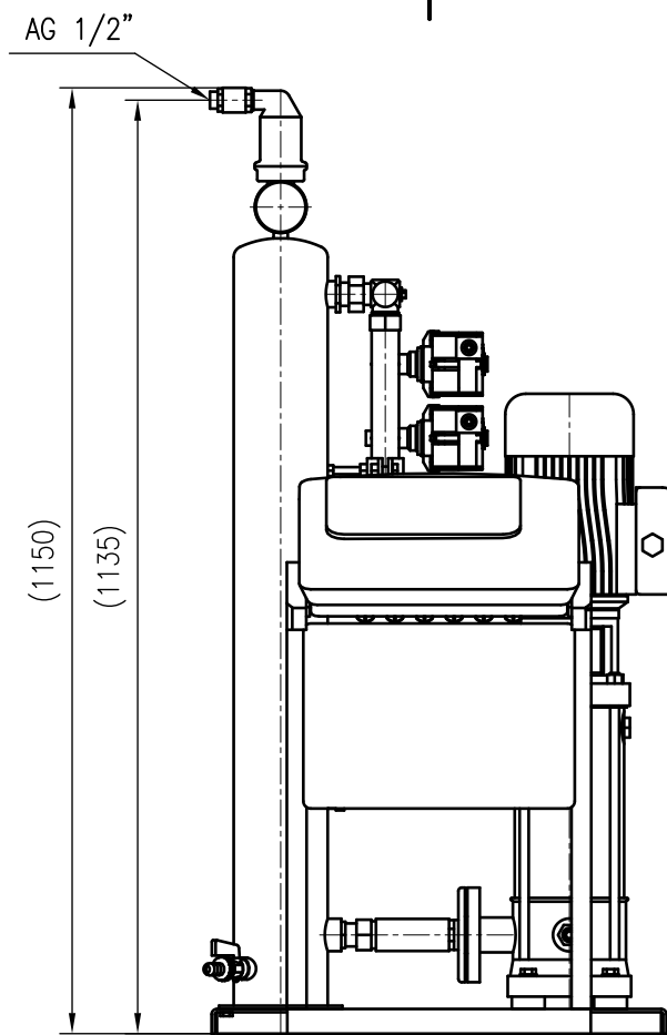
UNIDOMO® Front view
