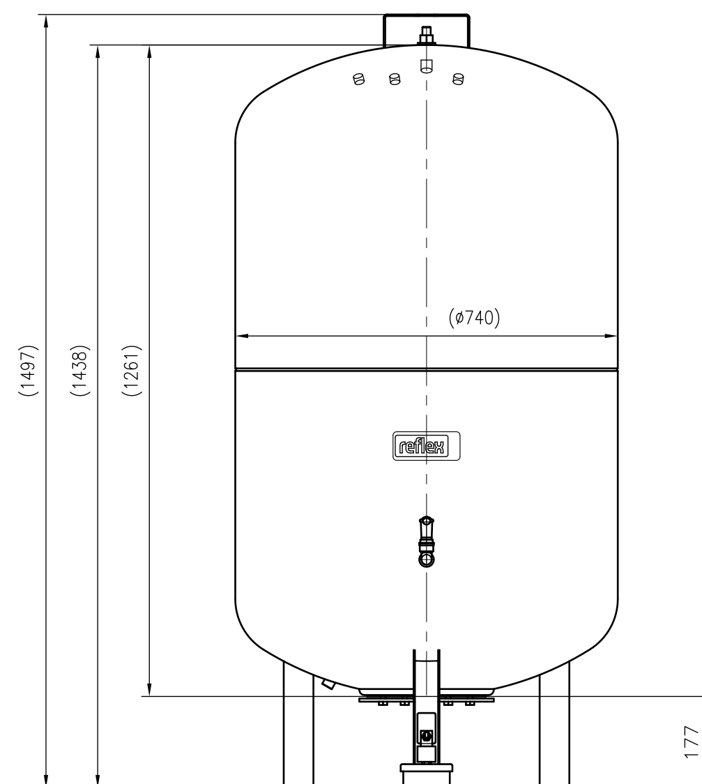
Front view UNIDOMO®
