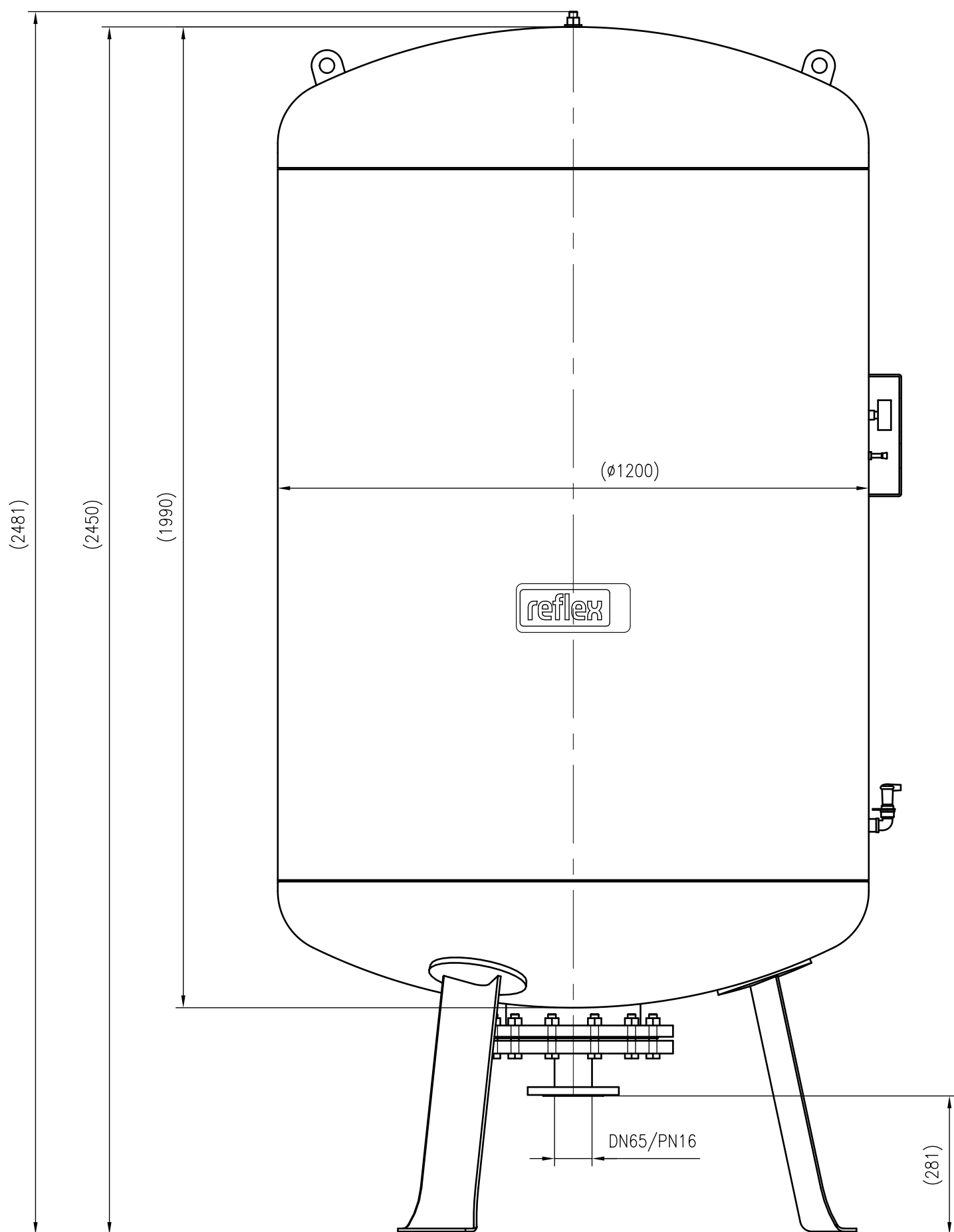
UNIDOMO® Front view
