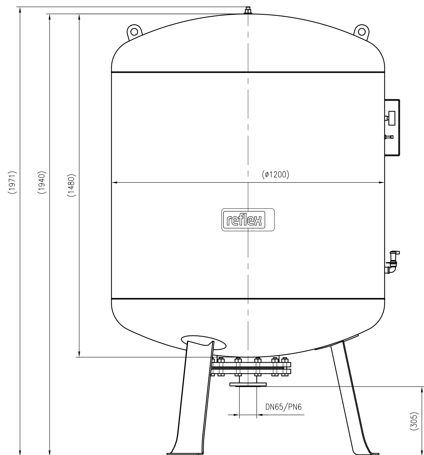
UNIDOMO® Front view
