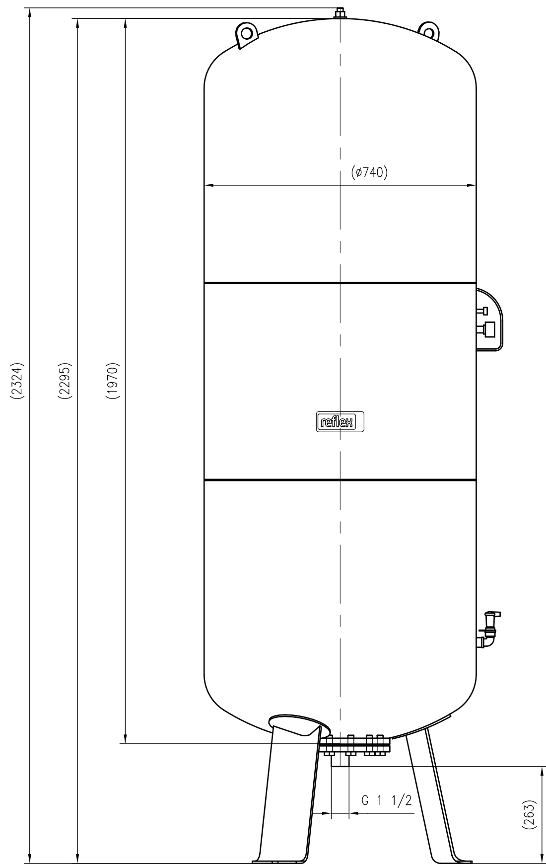
UNIDOMO® Front view
