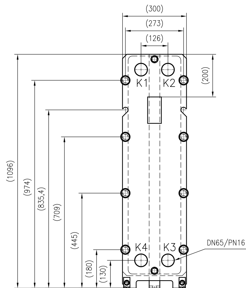
UNIDOMO® Front view
