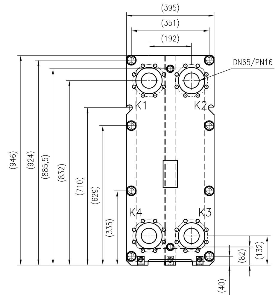
UNIDOMO® Front view
