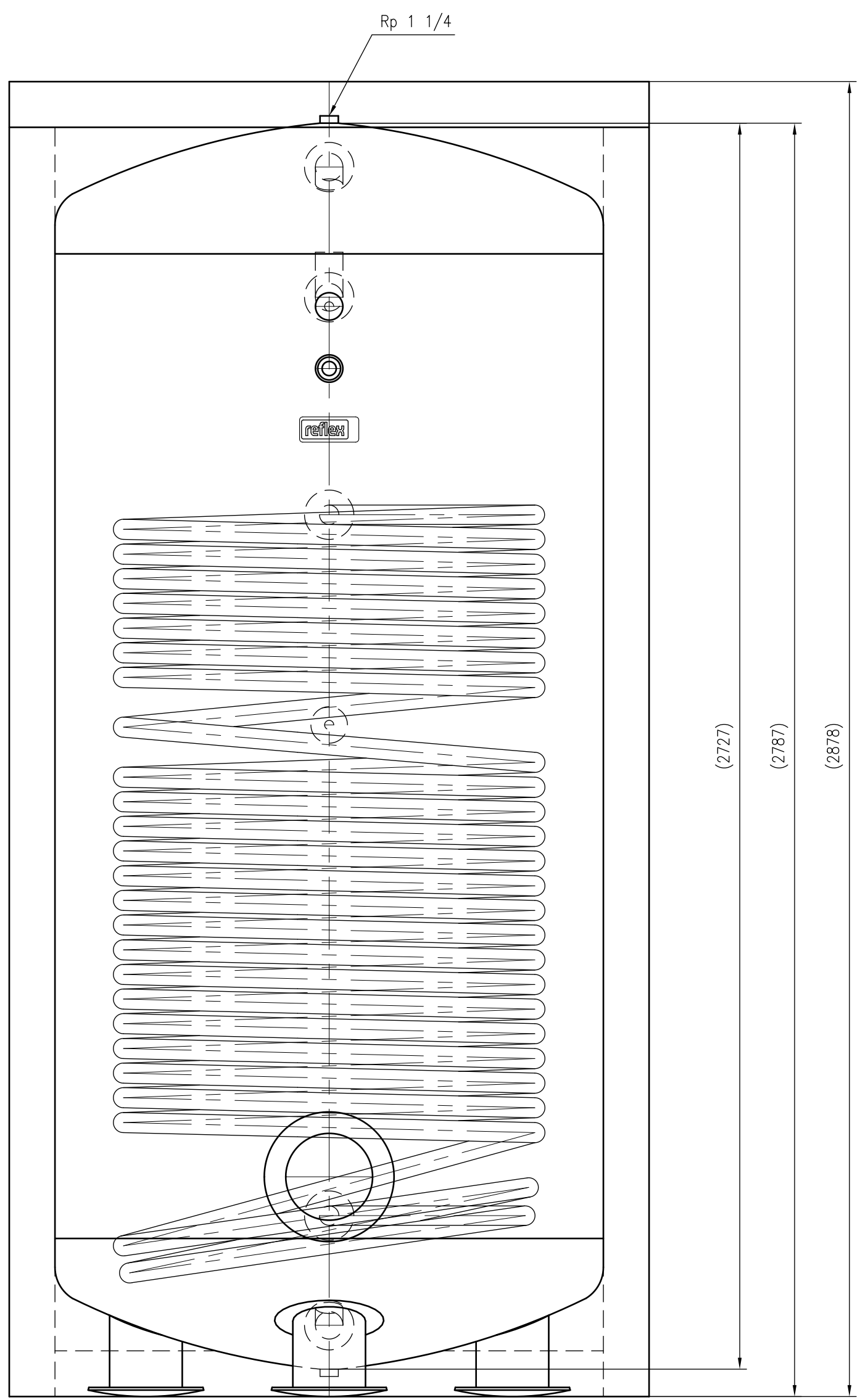
UNIDOMO® Front view
