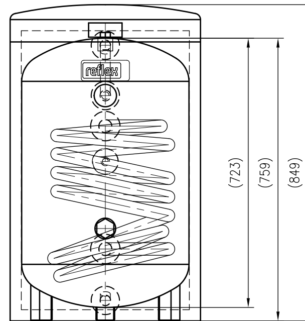
UNIDOMO® Front view
