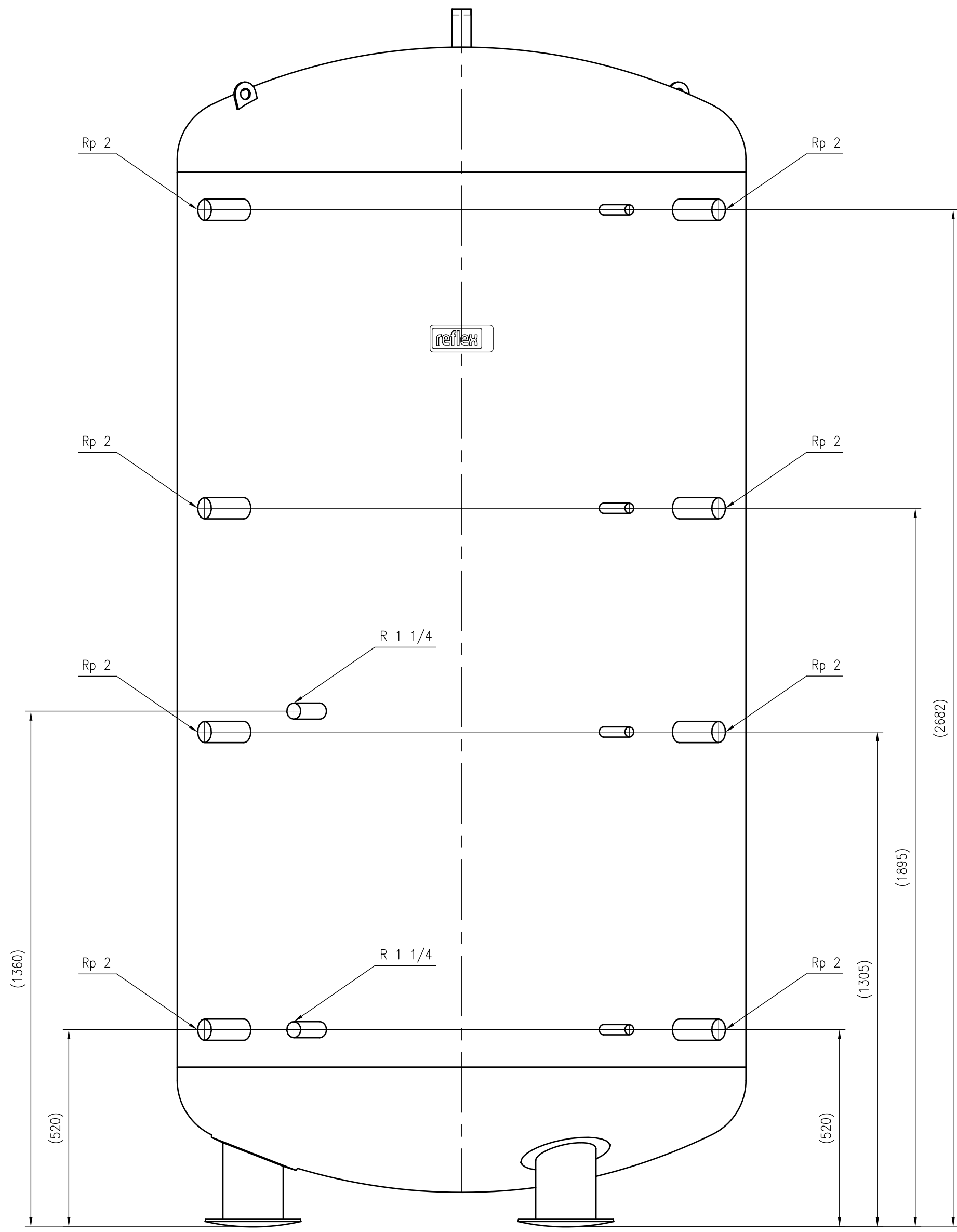
UNIDOMO® Front view
