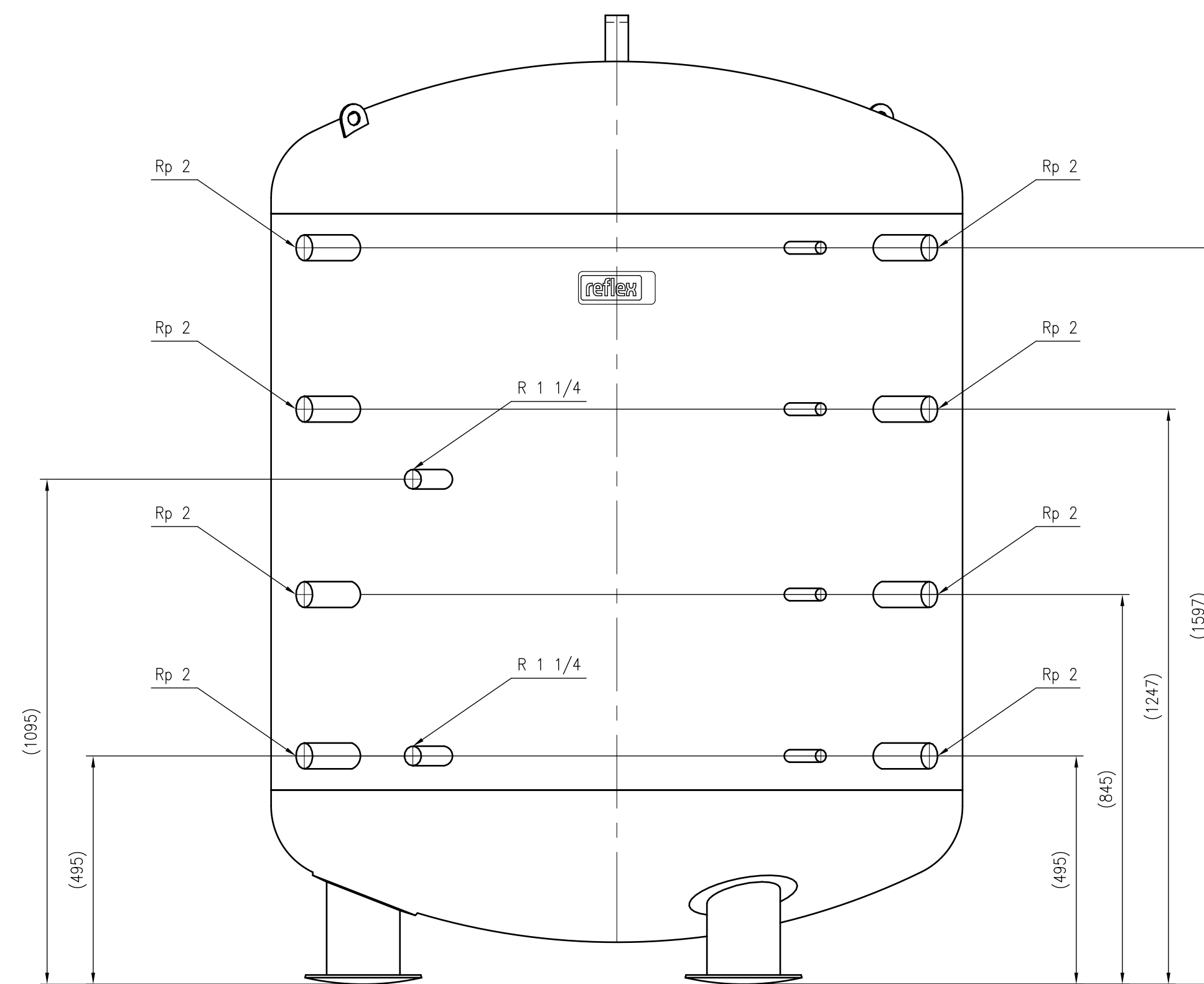
UNIDOMO® Front view
