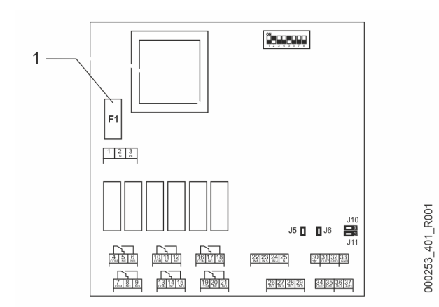
1 Precīzais drošinātājs F1 (250 V, 0, 16 A, inerts)
