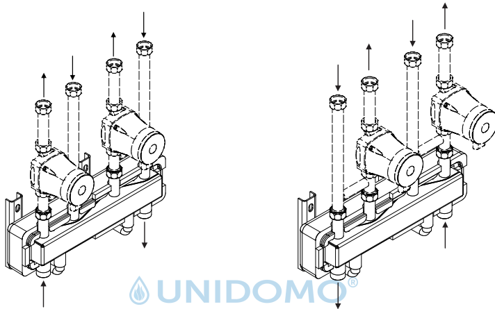
Für 2 / 4 / 6 ... Heizkreise / For 2 / 4 / 6 ... heating circuits
