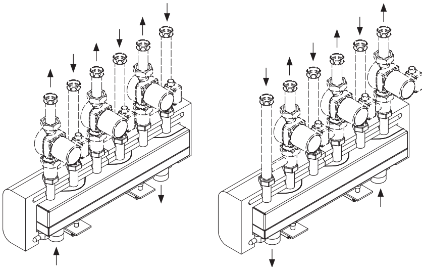
Für 3 / 5 / 7 ... Heizkreise / For 3 / 5 / 7 ... heating circuits
